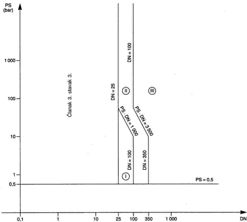
Dijagram 6. Cjevovodi iz članka 3. stavka 1. točke 3a, prva alineja
