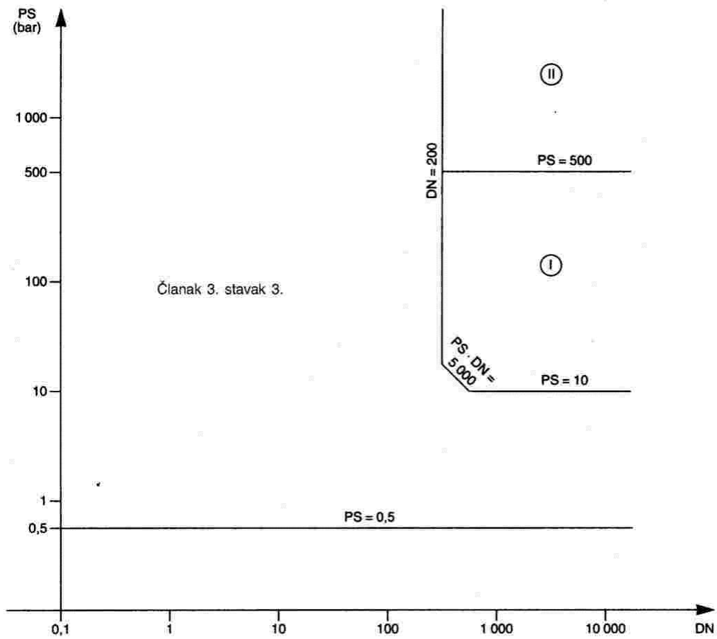
Dijagram 9. Cjevovodi iz članka 3. stavka 1. točke 3b, druga alineja
