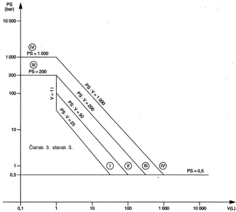
Dijagram 1. Posude iz članka 3. stavka 1. točke 1a, prva alineja
